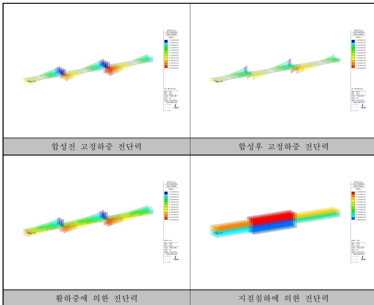
&lt;그림 5.6&gt; 구조해석에 의한 전단력 산출 결과
